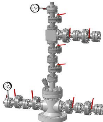
АФК2(Ш)-65х21 К1(К2)М4
